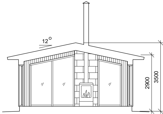
Sektion A-A Skala 1:100
