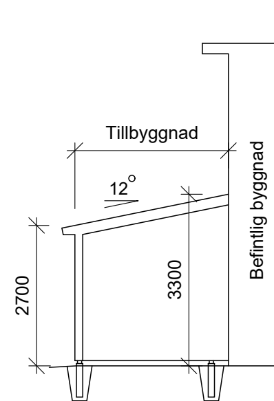
Sektion A-A
