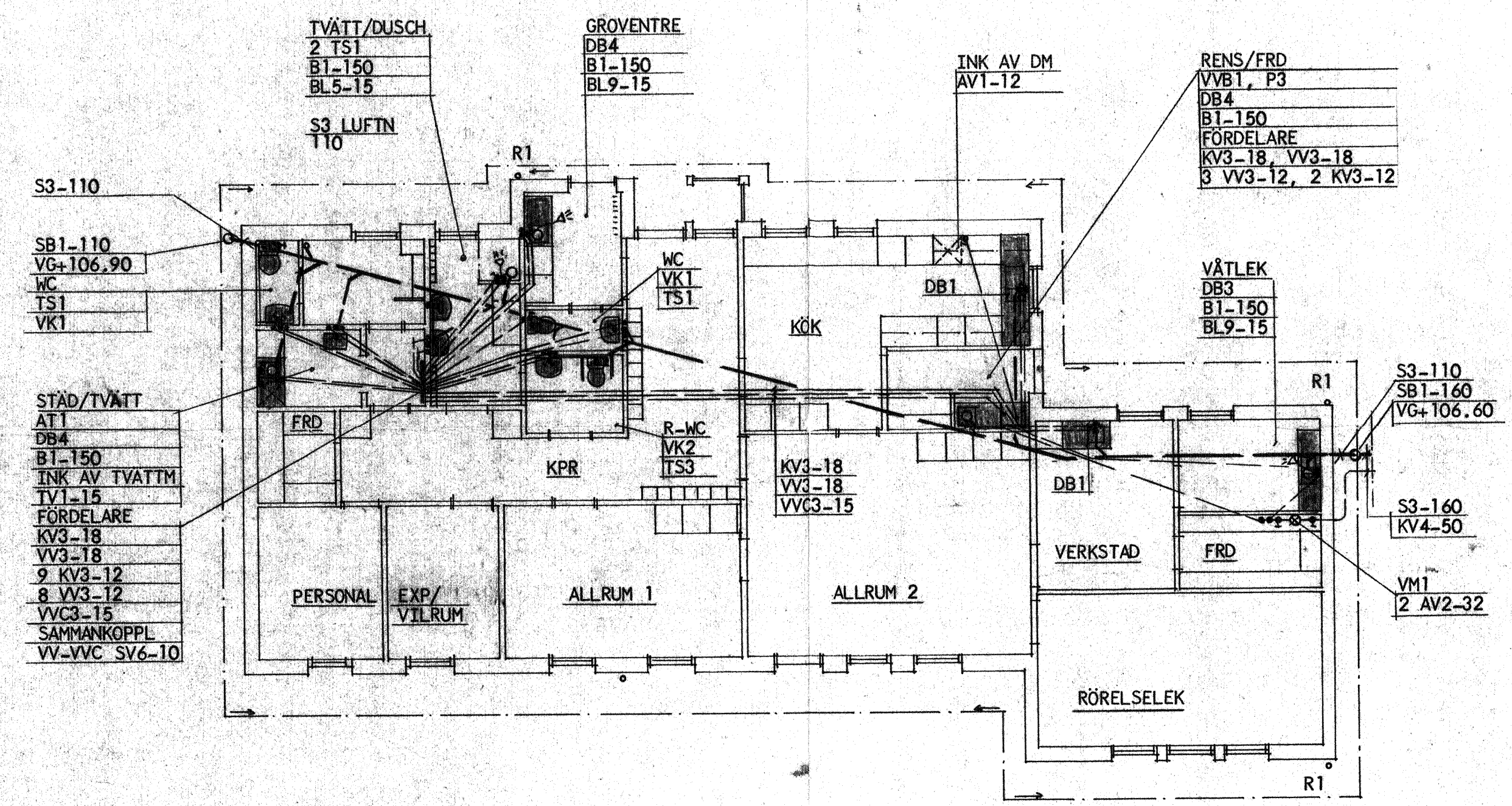
BOTTENPLAN 1:100
