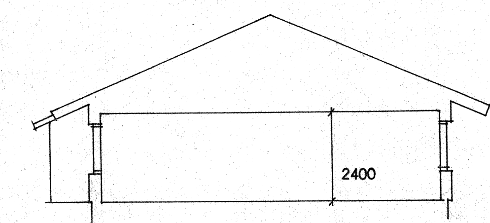
SEKTION 1:100
